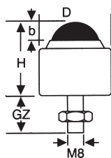
Rolle mit Gewindezapfen
