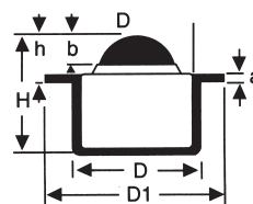
Rolle mit versenktem Gehäuse
